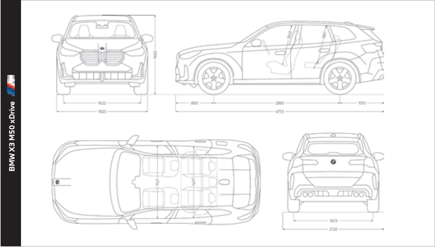
Toutes les cotes des dessins techniques sont indiquées en mm.
