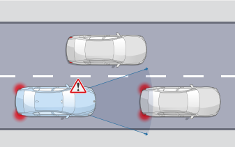
Avertisseur de collision frontale avec intervention de freinage
