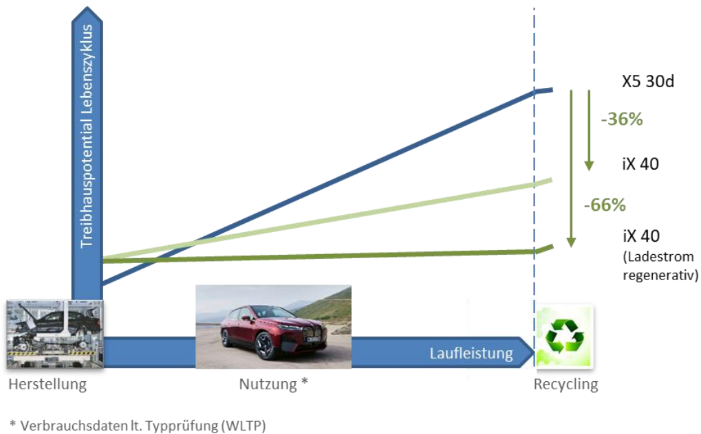
Abb. 3: Einordnung des BMW iX 40 in Bezug auf ein konventionelles Fahrzeugkonzept (X5 30d)
